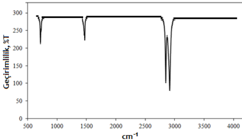
Şekil 2. Çözündürme sonrası geri kalan plastic malzemeye ait FT-IR analizi.
