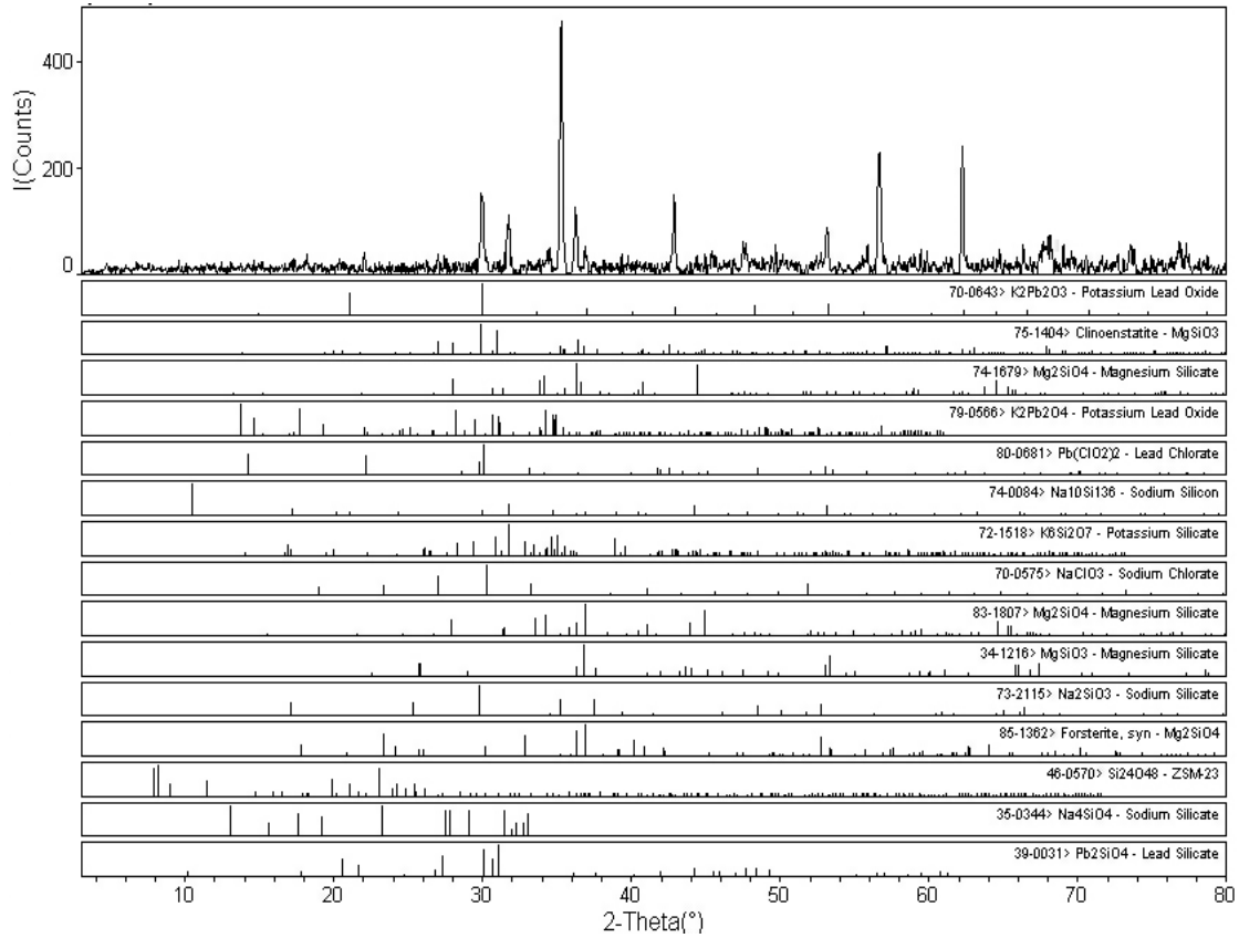
Şekil 1. Kurşun baca tozuna ait X-ışınları Kırınımı Difraksiyonu (XRD)
