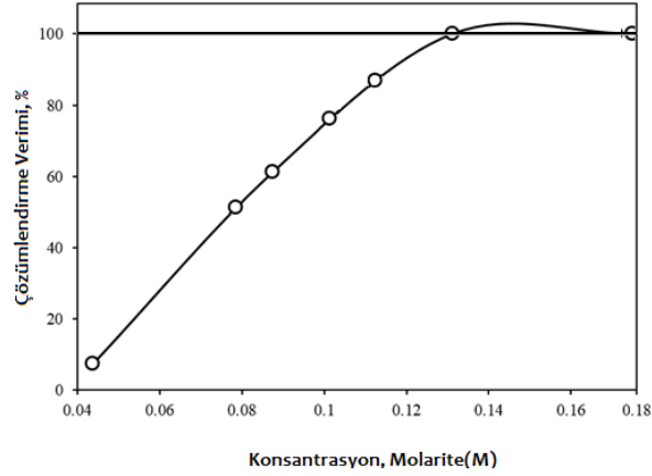
Şekil 1. Artan asit konsantrasyonuna karşı P-Al'nin çözündürme verimi.
