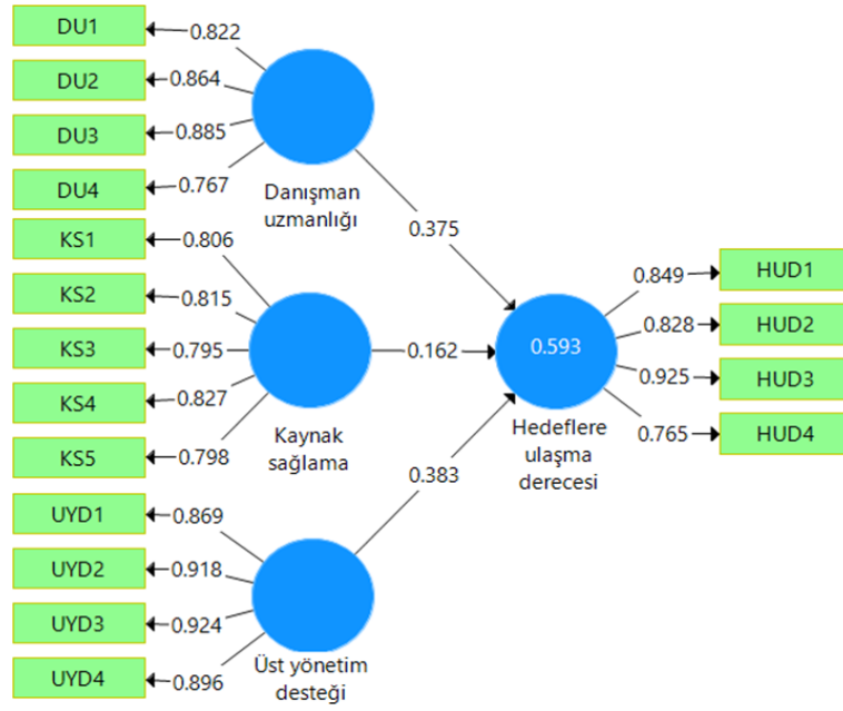
Şekil 3. KTGT Değişkenlerinin Hedeflere Ulaşma Derecesi Proje Başarısı Değişkenine Etkisine Yönelik Yol
