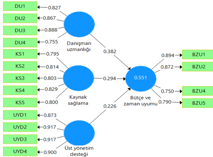
Şekil 2: KTGT Değişkenlerinin Bütçe ve Zaman Uyumu Proje Başarısı Değişkenine Etkisine Yönelik Yol
