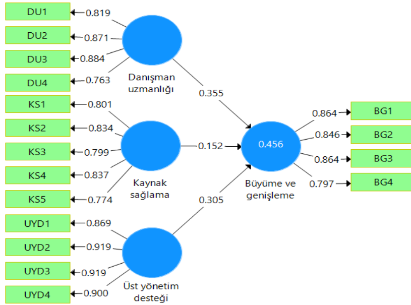
Şekil 5. KTGT Değişkenlerinin Büyüme ve Genişleme Proje Başarısı Değişkenine Etkisine Yönelik Yol Grafiği
