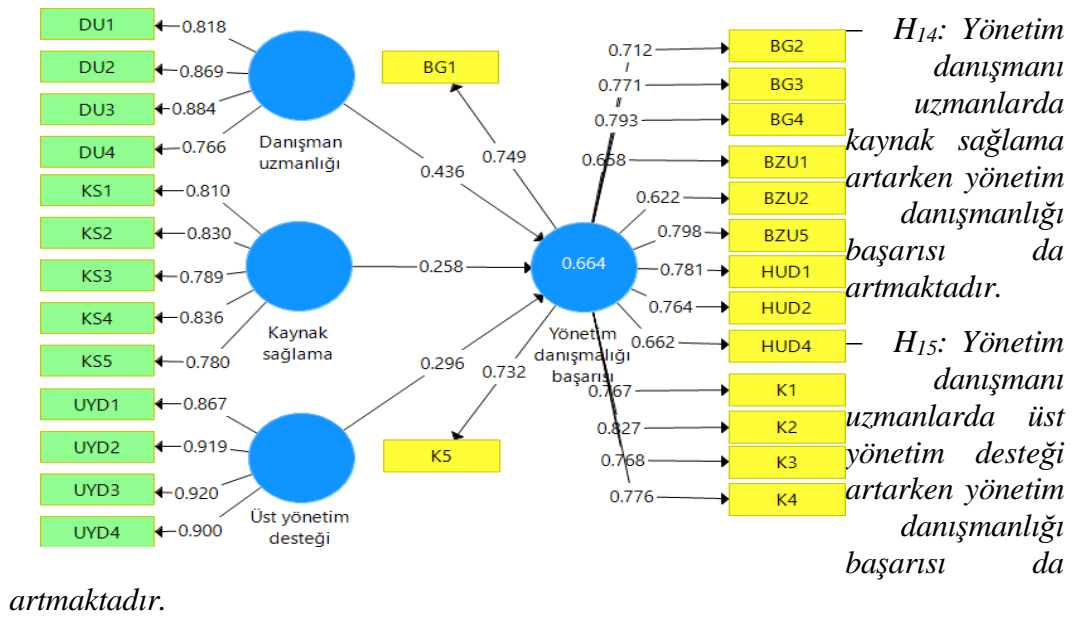
Şekil 6. KTGT Değişkenlerinin Yönetim Danışmanlığı Proje Başarısı Değişkenine Etkisine Yönelik Yol Grafiği
