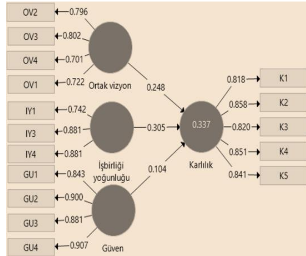
Şekil 4: AVT değişkenlerinin kârlılık proje başarısı değişkenine etkisine yönelik yol
