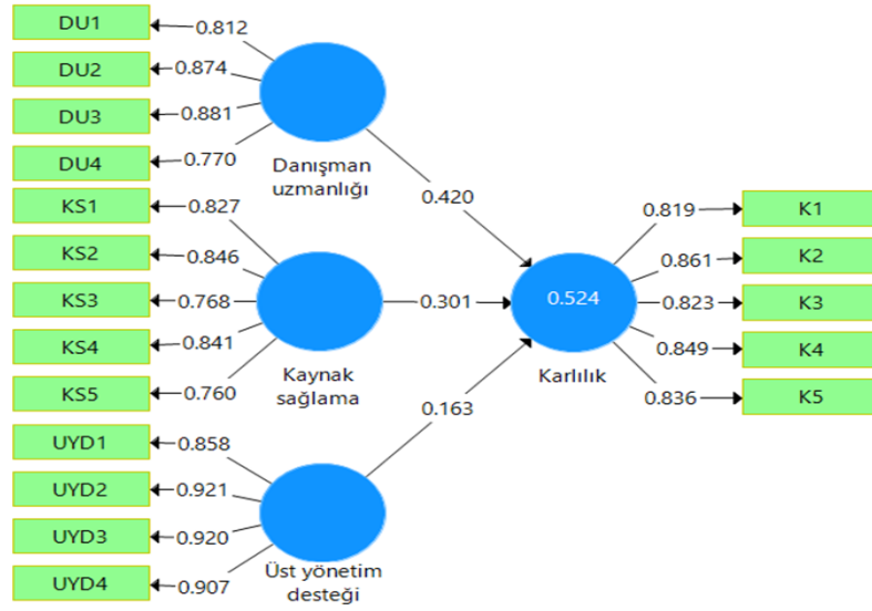
Şekil 4. KTGT Değişkenlerinin Kârlılık Proje Başarısı Değişkenine Etkisine Yönelik Yol
