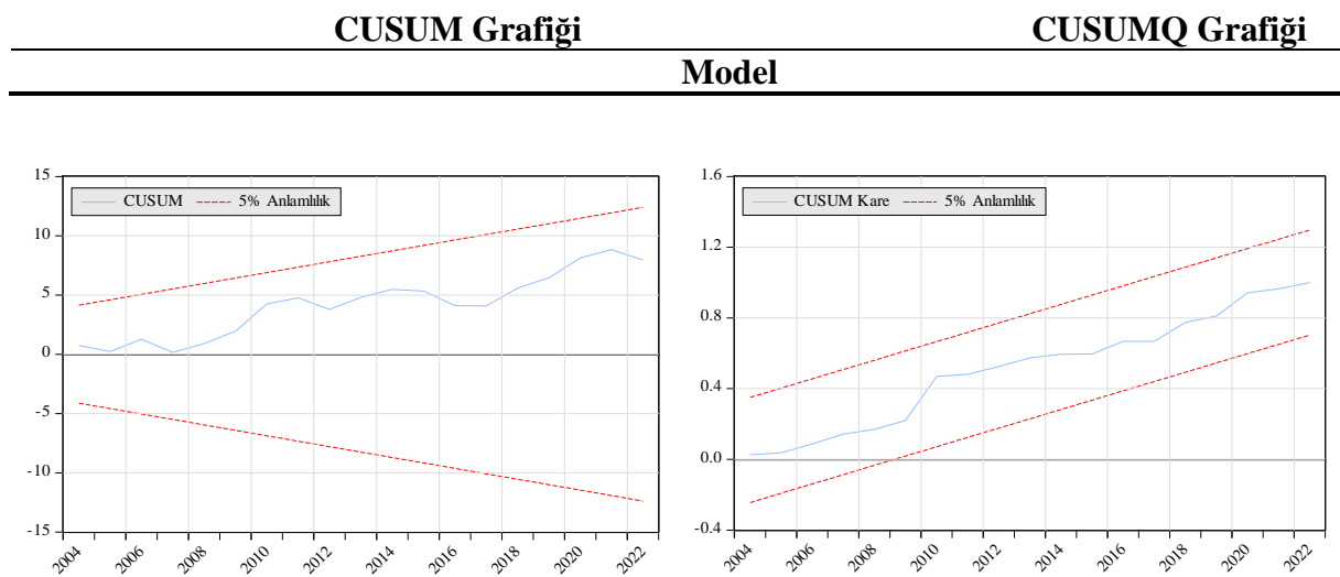
Grafik 3: Uzun Dönem Modellere Ait CUSUM ve CUSUMSQ Grafikleri
