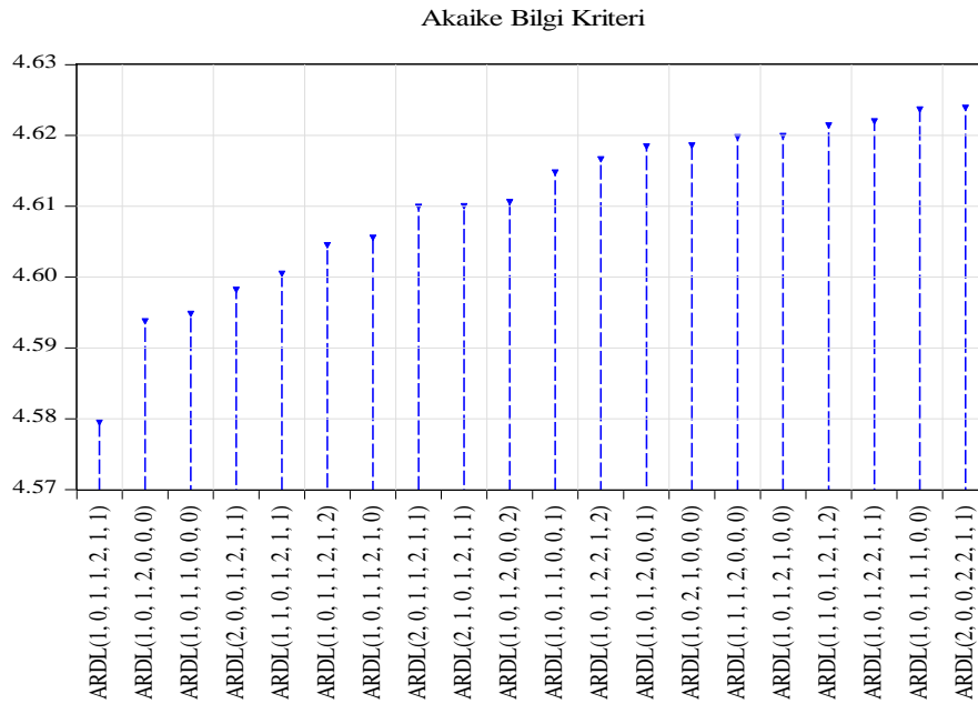
Grafik 2: Optimal Gecikme Seçimi için Akaike Bilgi Kriteri Karşılaştırmaları
