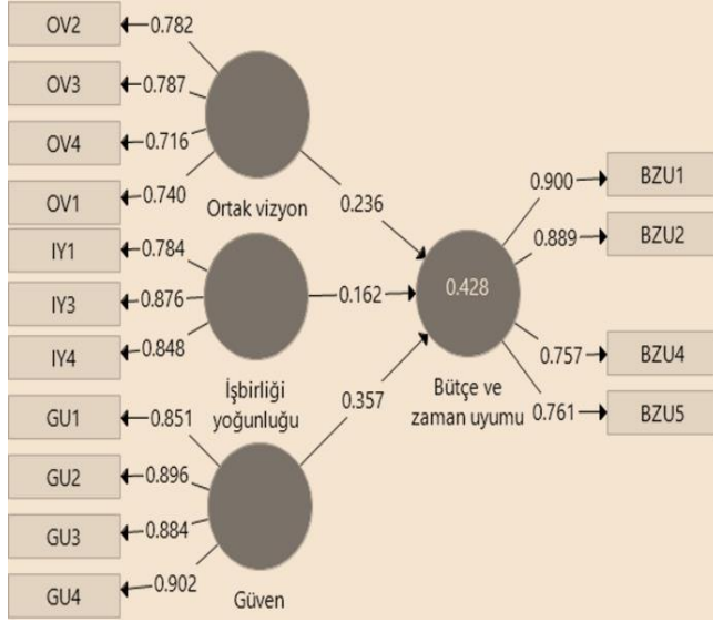
Şekil 2. Asil Vekil Teorisi değişkenlerinin "bütçe ve zaman uyumu" proje başarı değişkenine etkisine
