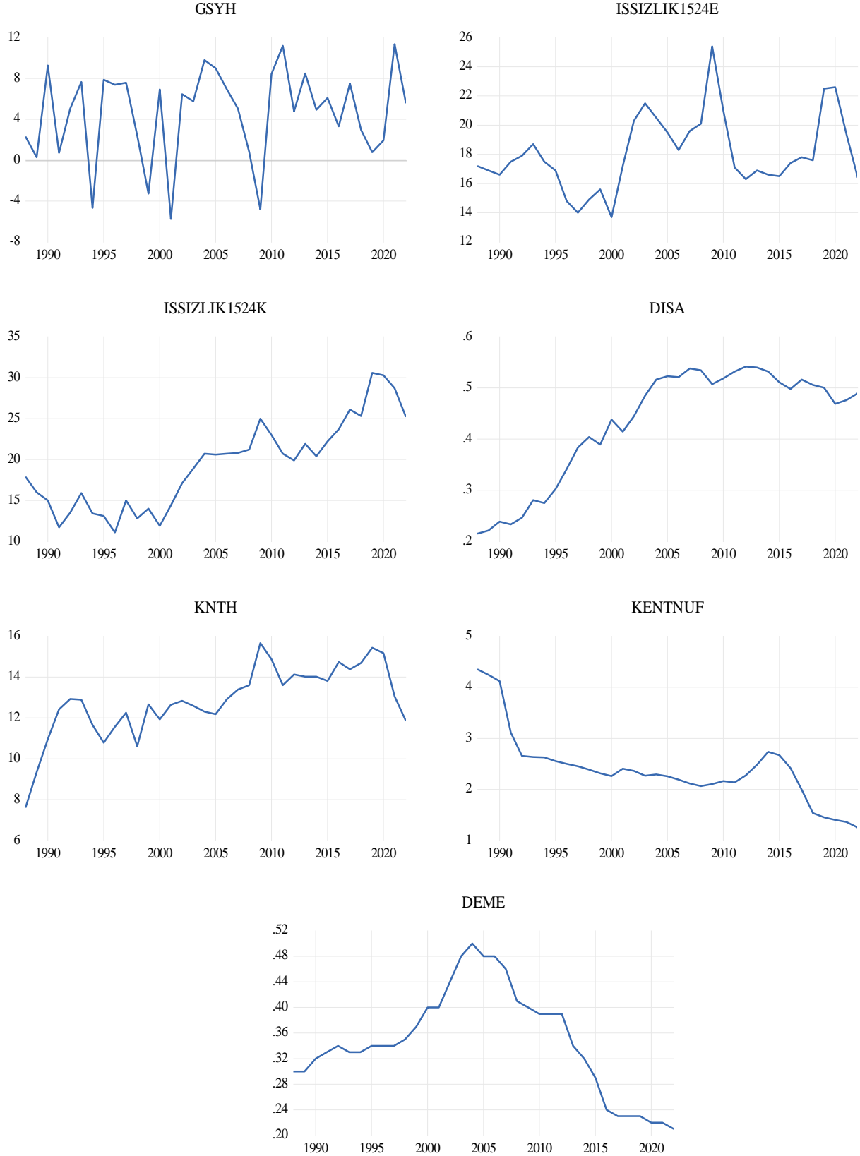
Grafik 1: Değişken Zaman Seyir Grafikleri
